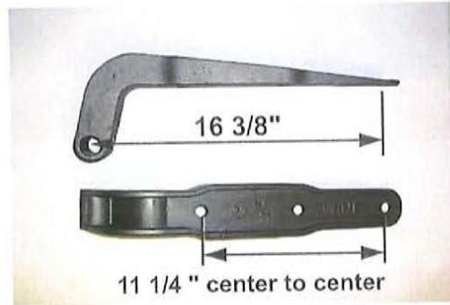
DA Part # : DA- 23261 Ref # : HF-261 Description: HINGE
