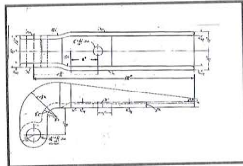
DA Part # : DA- 45496 Ref # : MC-496 Description: HINGE
